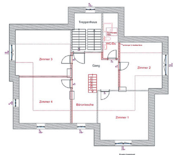
Projektpläne 3. Obergeschoss Pfarrhaus
